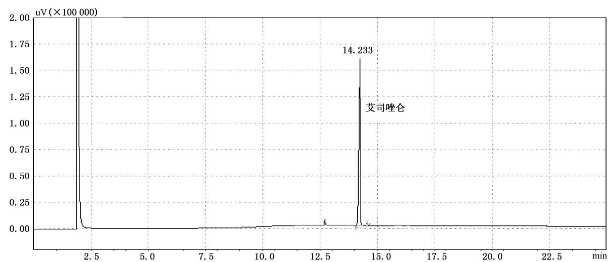
图 B.1 艾司唑仑气相色谱图
