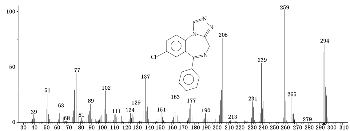
图 B.2 艾司唑仑质谱图
